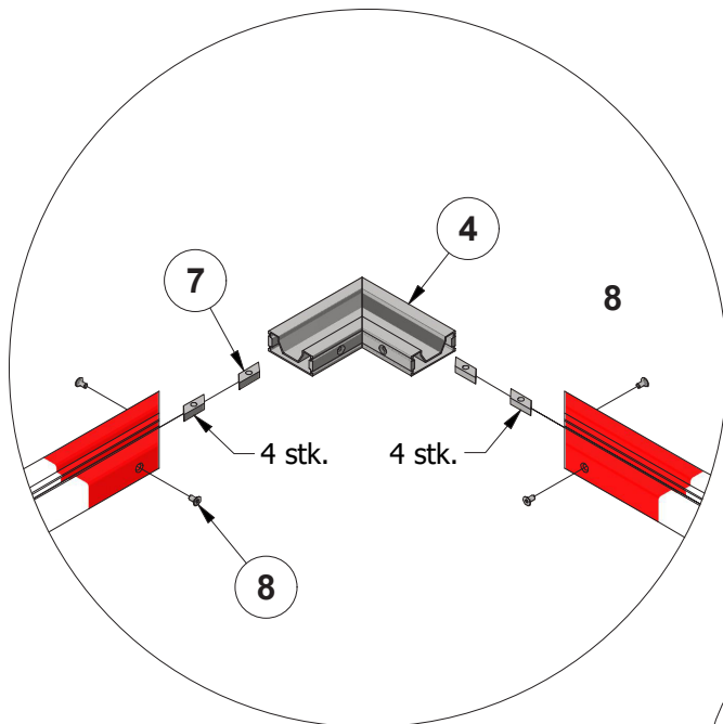
A ( 1 : 10 )
